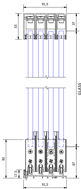
Система 4 панела
