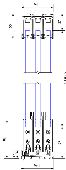
Система 3 панела
