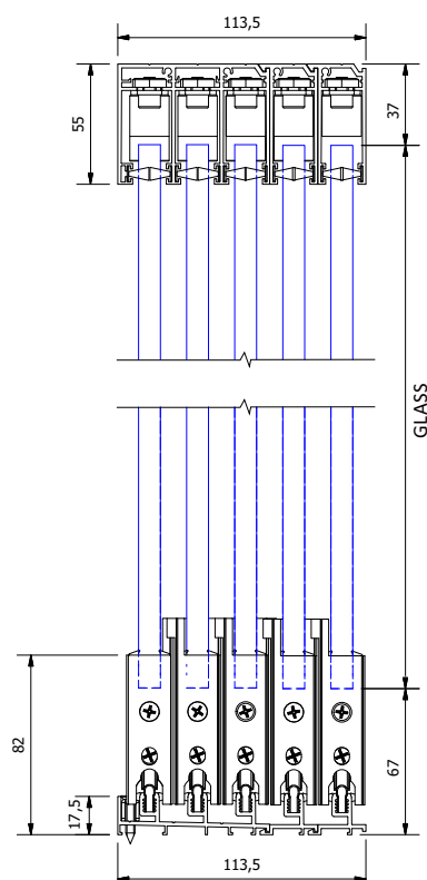
Система 5 панела
