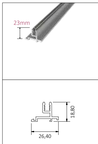
Единична релса
